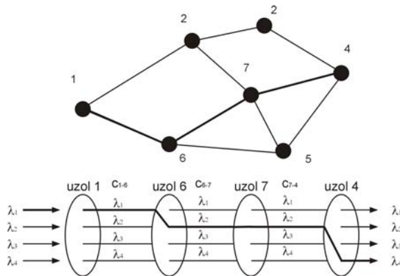
Obr. 3 Smerovanie a prideľovanie vlnovej dĺžky Fig. 3 Routing and wavelength assignment
